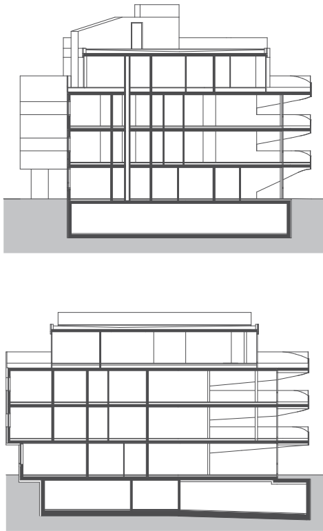
SCHNITTE
